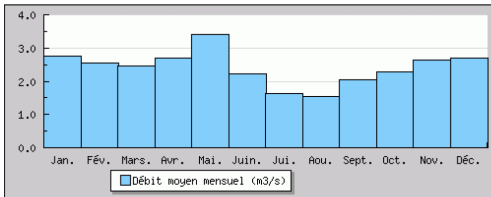
Illustration III.5: Hydrogramme du Furan à Andrézieux-Bouthéon/Banque Hydro
