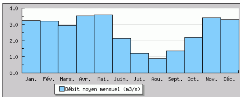
Illustration III.3: Hydrogramme du Gier à la station Rive de Gier / Banque Hydro
